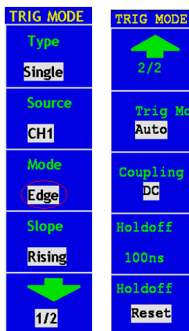
Fig. 44 Edge trigger menu
