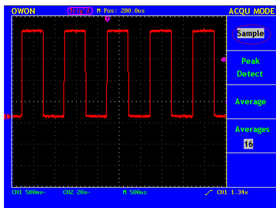
Fig. 54 Normal ACQU Mode
