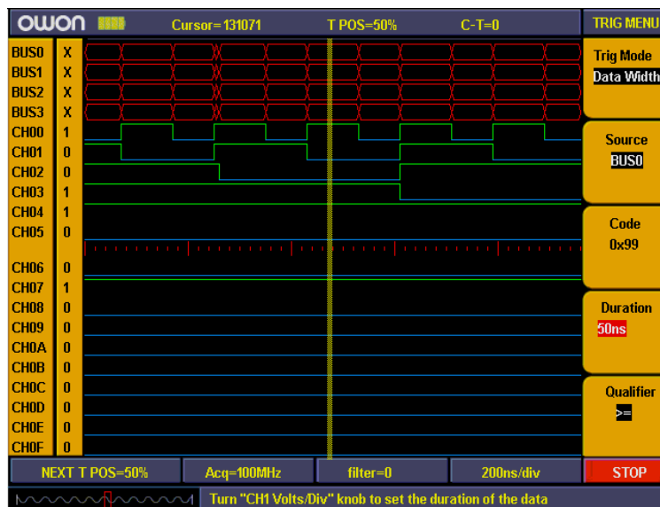
Fig. 91: Data width trigger
