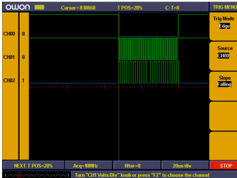
Fig.81: Edge trigger setting
