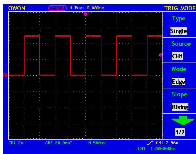
Fig.4 Auto set
